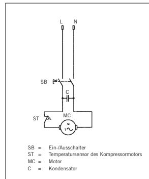
Schaltplan ha 1000, 230 V
